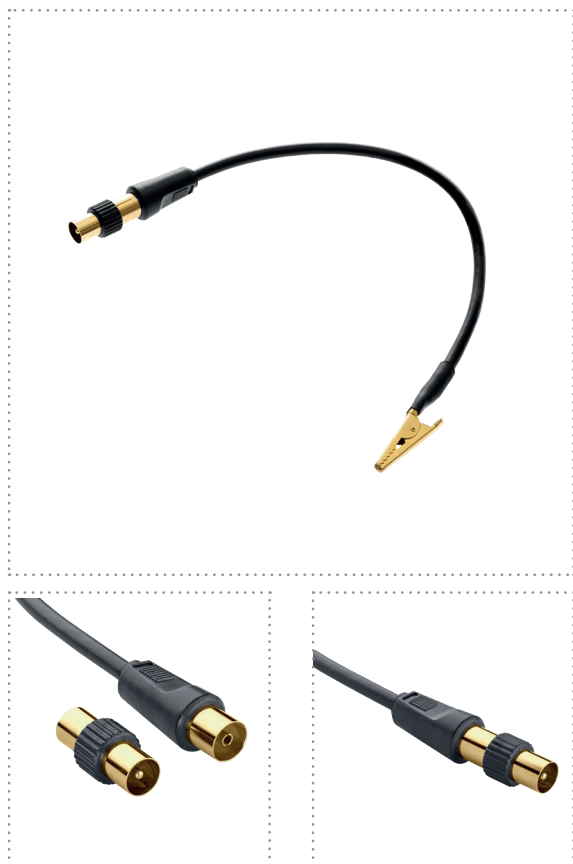
Fiche d'antenne mâle Pince crocodile
